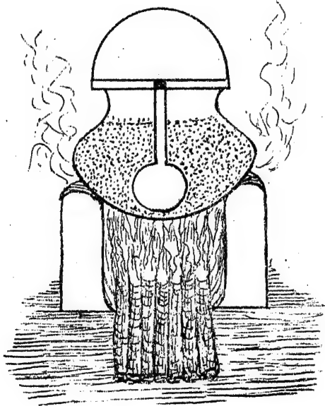
वालुकायन्त्रम् १३
